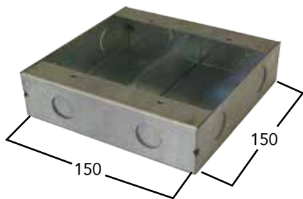
Conduit Box Pre-Galvanised
